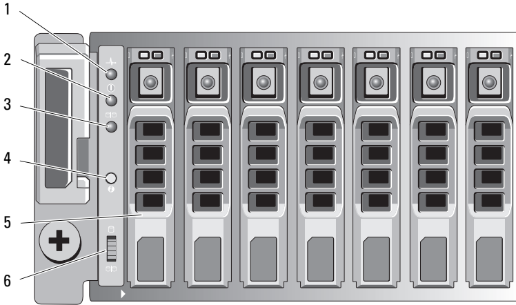
图 2-2. 前面板部件和指示灯 — Dell PowerVault MD3620f
